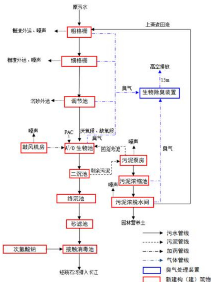
图 3.1-5 污水处理工艺流程及产污环节图
