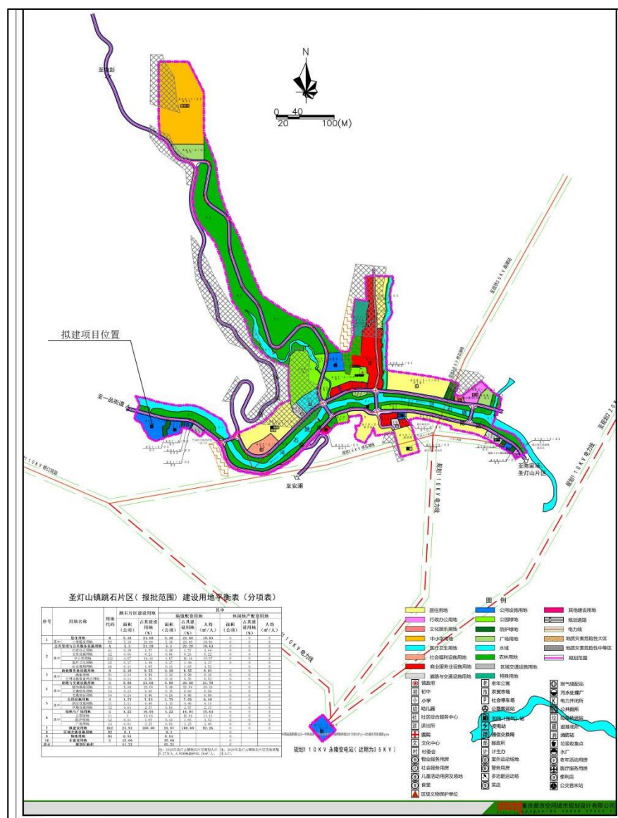
图 3.1-1 圣灯山镇污水厂服务范围图（紫红色区域）
